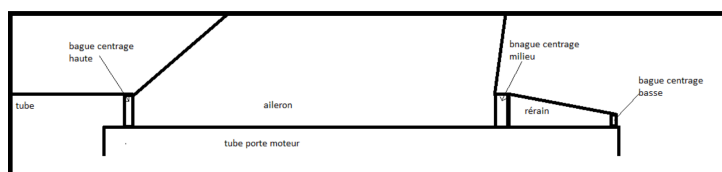
FIGURE 4.1 – Procédé de collage ailerons/tube porte-moteur
